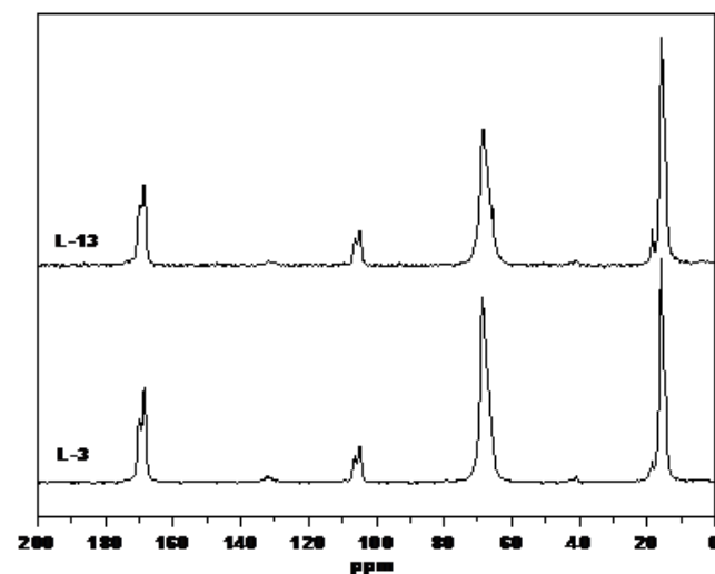
Fig.5. 13 C CP/MAS (300 MHz) L-3 and L-13.
